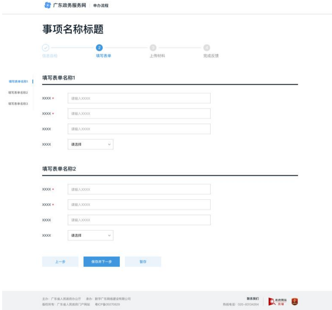
图23 填写表单页
