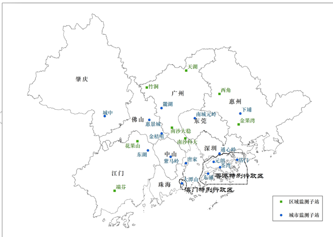
图 2.1: 粤港澳珠江三角洲区域空气监测网络子站的空间分布图 2
