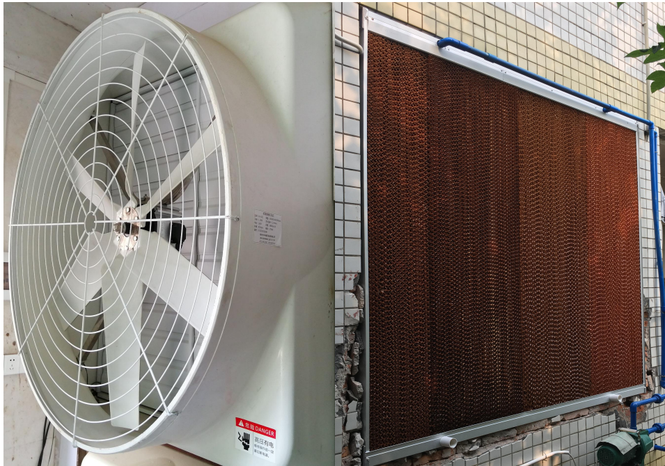
9SLJ-2000×2000×150 型水帘降温设备
